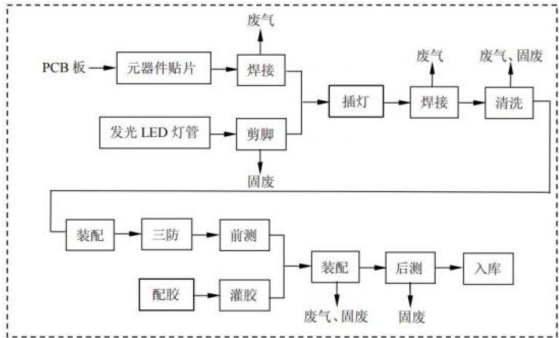
图 1-2 直插模块加工生产工艺流程图
