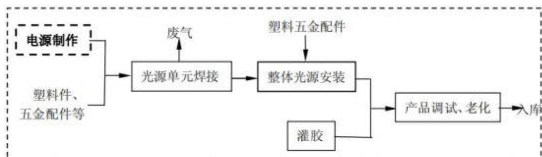
图 1-5 LED 照明灯生产工艺流程图
