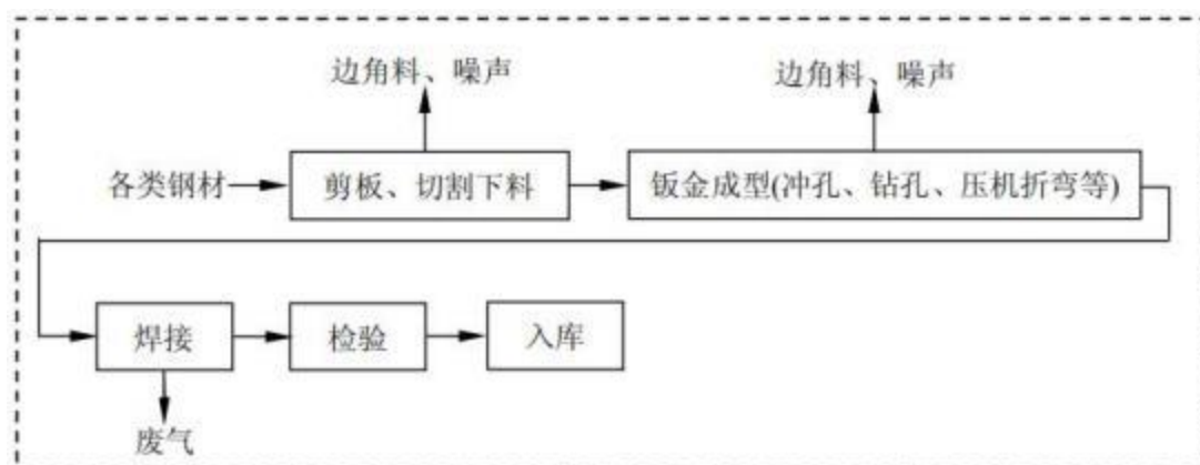
图 1-8 金属配件生产工艺流程图
