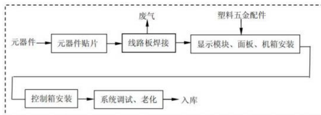
图 1-4 LED 显示屏生产工艺流程图
