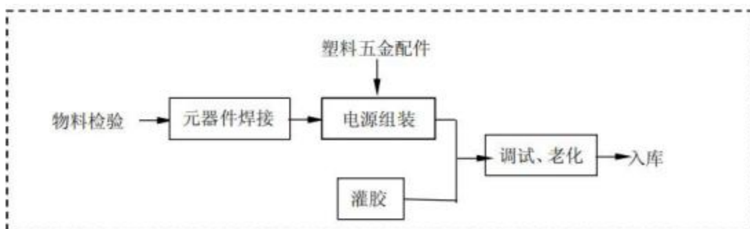
图 1-6 电源制作工艺流程图
