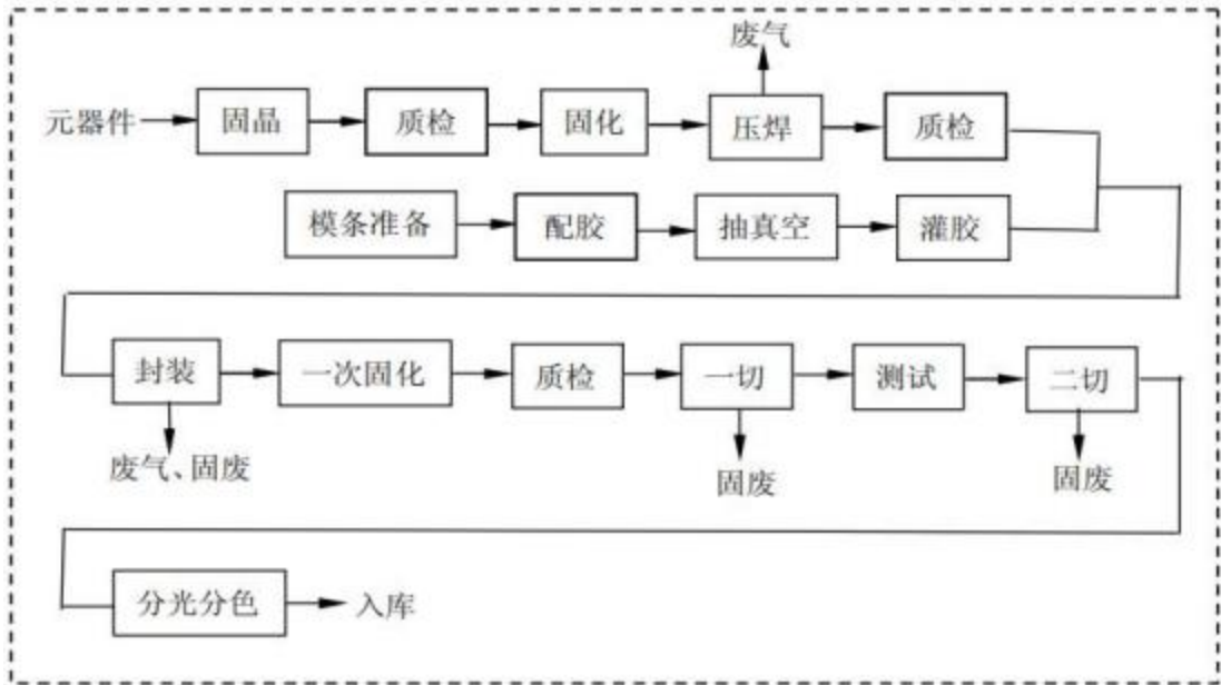
图 1-1 直插灯封装生产工艺流程图
