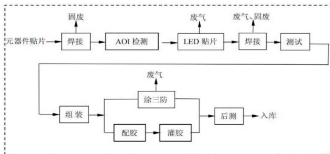
图 1-3 表贴模块加工生产工艺流程图
