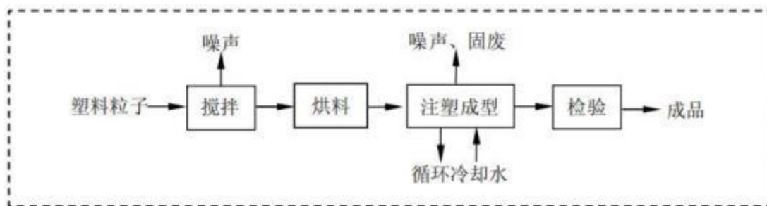
图 1-7 塑料配件生产工艺流程图
